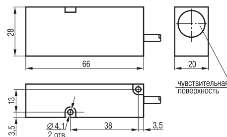
Габаритный чертеж
