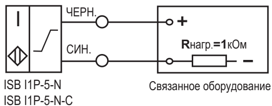
Схема подключения к оборудованию
